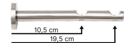
A Podwójny profilowy Double profile
