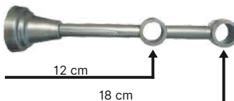
A Podwójny Leon Double Leon
